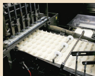
全自動餃子製造機
